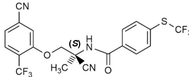
MONEPANTEL
